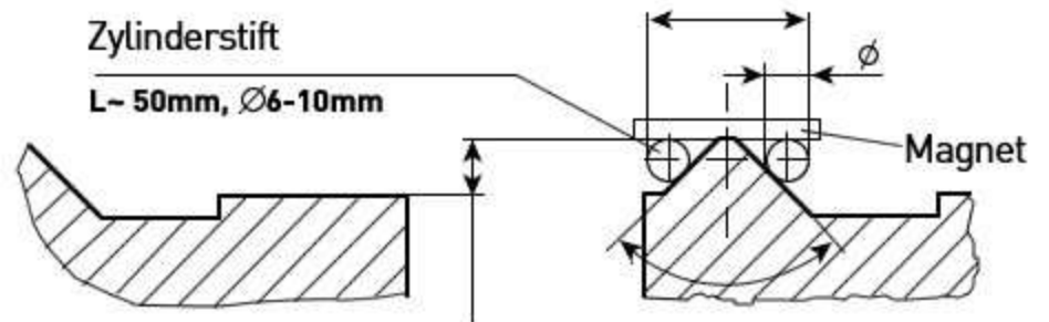
Empfehlungsschema für genaues Abmessen des Reitstockprismas
