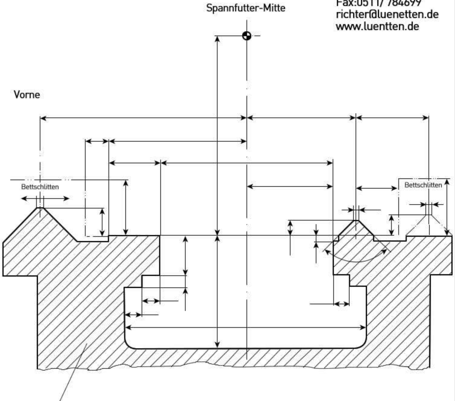
Empfehlungsschema für genaues Abmessen des Reitstockprismas
